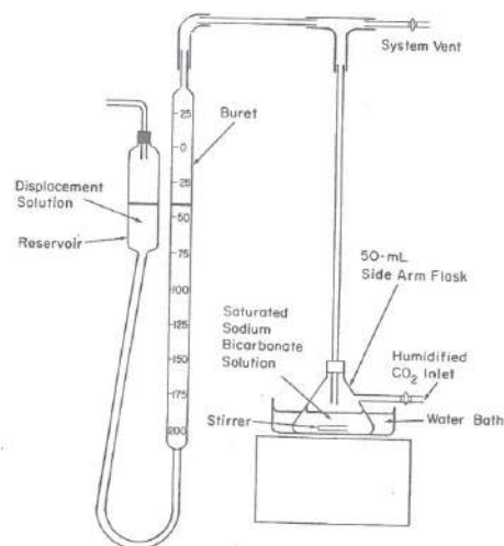
Carbonate Apparatus
